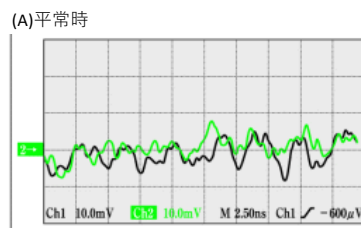
約2.0mV～8.0mVの電圧がZEROの回路に常に流れています。 【使用前】
